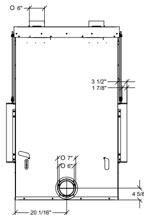
Vue arrière
