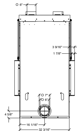
Vue arrière
