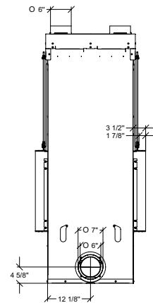
Vue arrière
