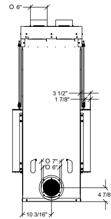
Vue arrière
