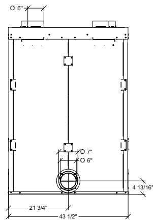
Vue arrière
