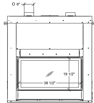
Vue arrière
