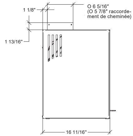
Vue latérale
