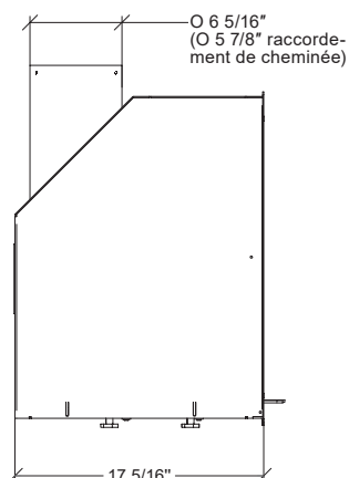
Vue latérale
