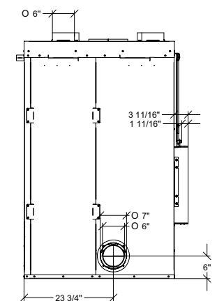
Vue arrière
