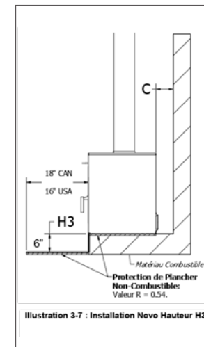
Illustration 3-7 : Installation Novo Hauteur H3
