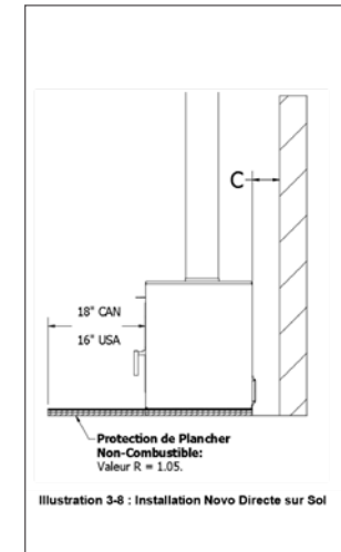
Illustration 3-8 : Installation Novo Directe sur Sol
