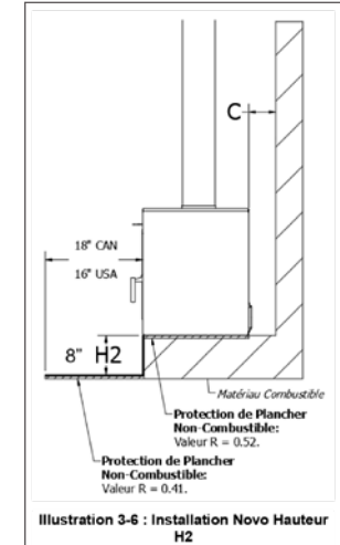
Illustration 3-6 : Installation Novo Hauteur H2
