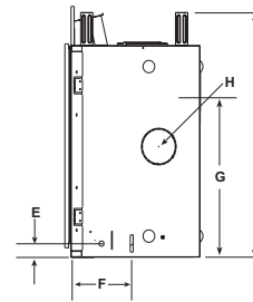
VUE LATÉRALE DROITE
